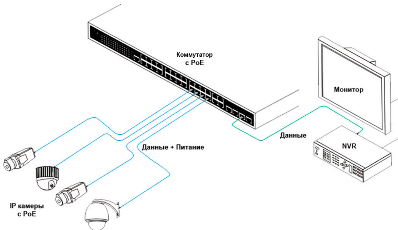
Рис. 3. Схема подключения
